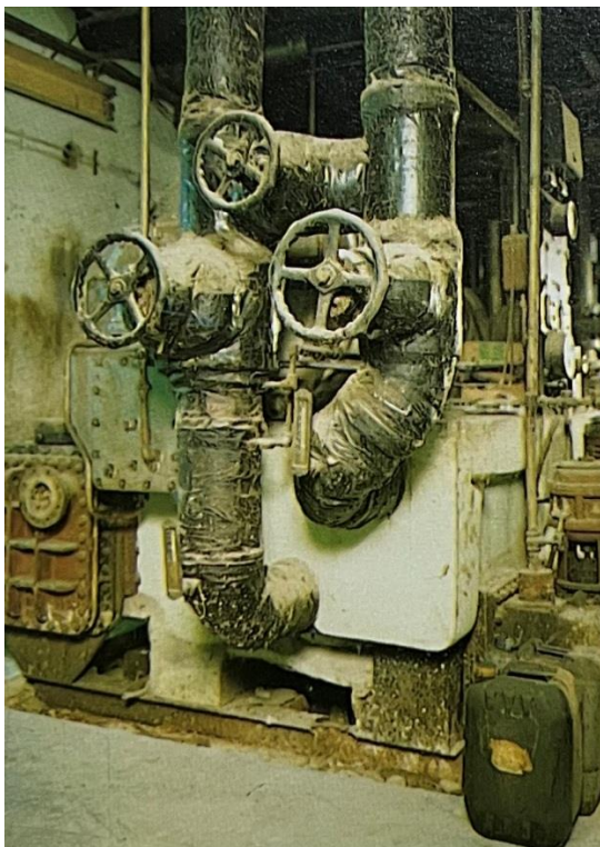
ภาพที่ 5 เครื่องปรับอากาศระบบไอน้ำ เครื่องแรกของประเทศไทย ที่มา : บริษัท เอลิมกรุ๊ปมณีทัศน์ จำกัด, ศาลาเฉลิมกรุง, 2537, 124
