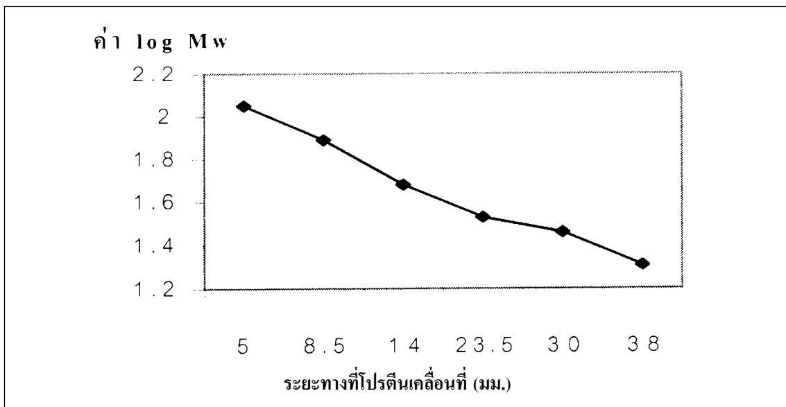
รูปที่ 1 กราฟความสัมพันธ์ระหว่างค่า log น้ำหนักโมเลกุลและระยะทางที่โปรตีนมาตรฐานเคลื่อนที่
