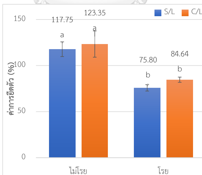
ภาพ 4.23 ค่าร้อยละการยืดตัว (percent elongation) ของแผ่นฟิล์มบรรจุรสน้ำยำที่คัดเลือกได้ 2 สูตร แบบไม่โรยพริกชี้ห์หุ่่น และแบบโรยพริกชี้ห์หุ่่น
