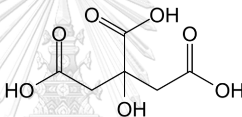
ภาพ 2.5 สูตรโครงสร้างของกรดซิตริก (citric acid)
