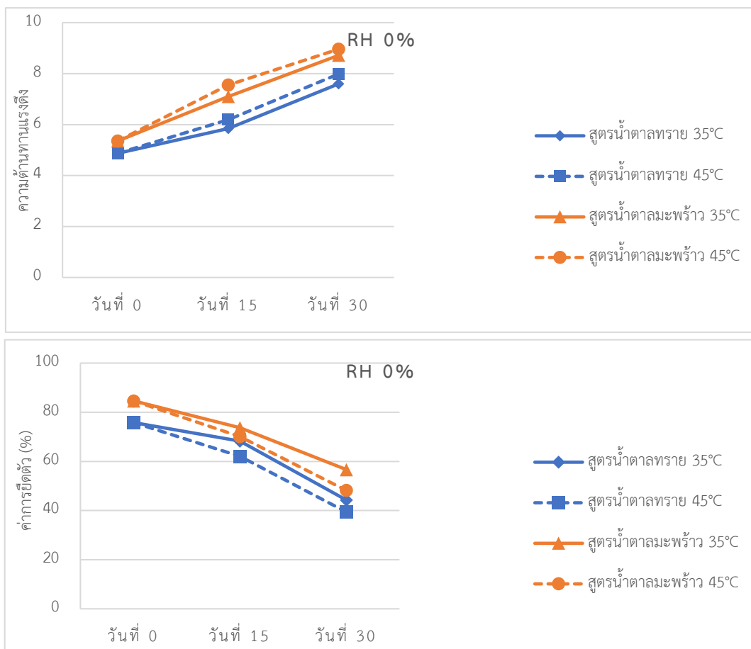
ภาพ 4.34 ค่าความต้านทานแรงดึง (tensile strength) และค่าร้อยละการยืดตัว (percent elongation) ที่ภาวะความชื้นสัมพัทธ์ที่ 0% ของแผ่นฟิล์มปรุงรสน้ำยำบรรจุในถุงพลาสติกพอลิโพรพิลีนปิดสนิทเก็บรักษาในที่มืดเป็นเวลา 30 วัน
