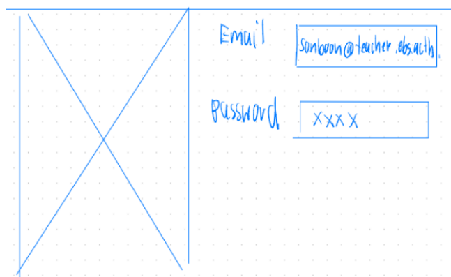
รูปที่ 4-52: ต้นแบบแบบหยาบหน้าการเข้าสู่ระบบ
